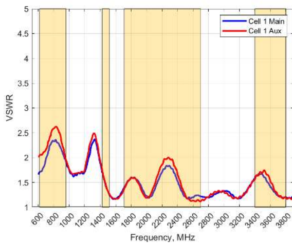
VSWR: Cell 1
