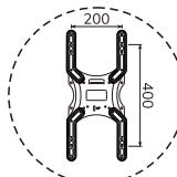
VESA 200x400
