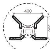
VESA 400x300
