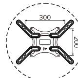
VESA 300x200
